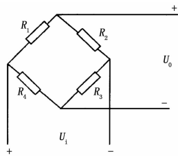
图 6 压力传感器原理图
