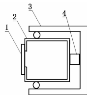
图 8 机架机械结构图
