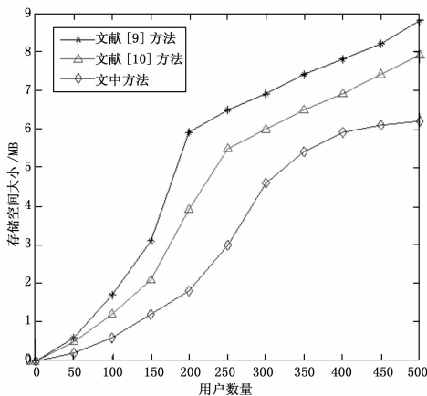
图 4 存储空间随用户个数变化比较
