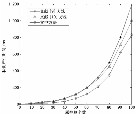
图 2 私钥产生时间随属性个数变化比较
