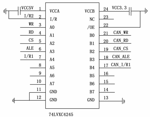
图 5 电平转换 74LVC4245 模块原理图
