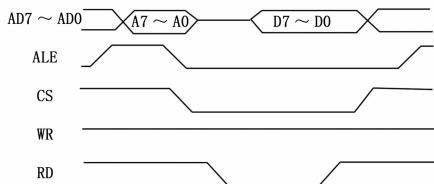
图 7 SJA1000 读时序
