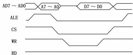
图 6 SJA1000 写时序
