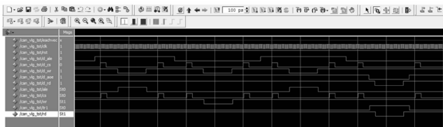
图 8 FPGA 模块程序仿真图
