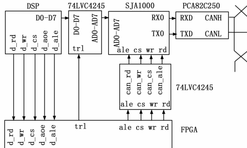
图 1 系统原理图
